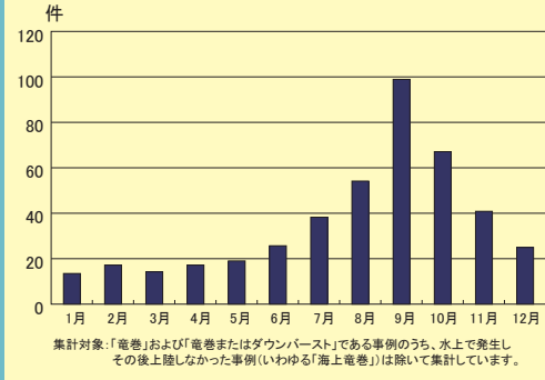
竜巻の月別発生確認数(1991～2015年)
