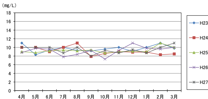
図 3.17 D0 の年間変動（金井沢橋）
