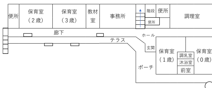
1階平面図
