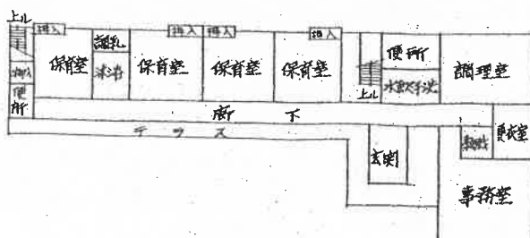
1 階平面図 S=1:400
