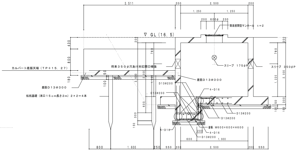
C-C 断面図
