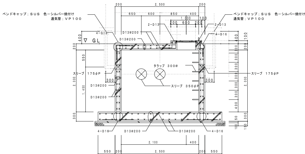
A-A 断面図
