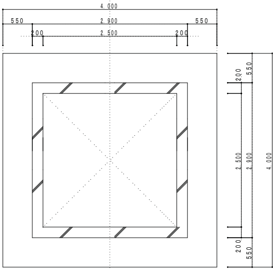
底盤平面図
