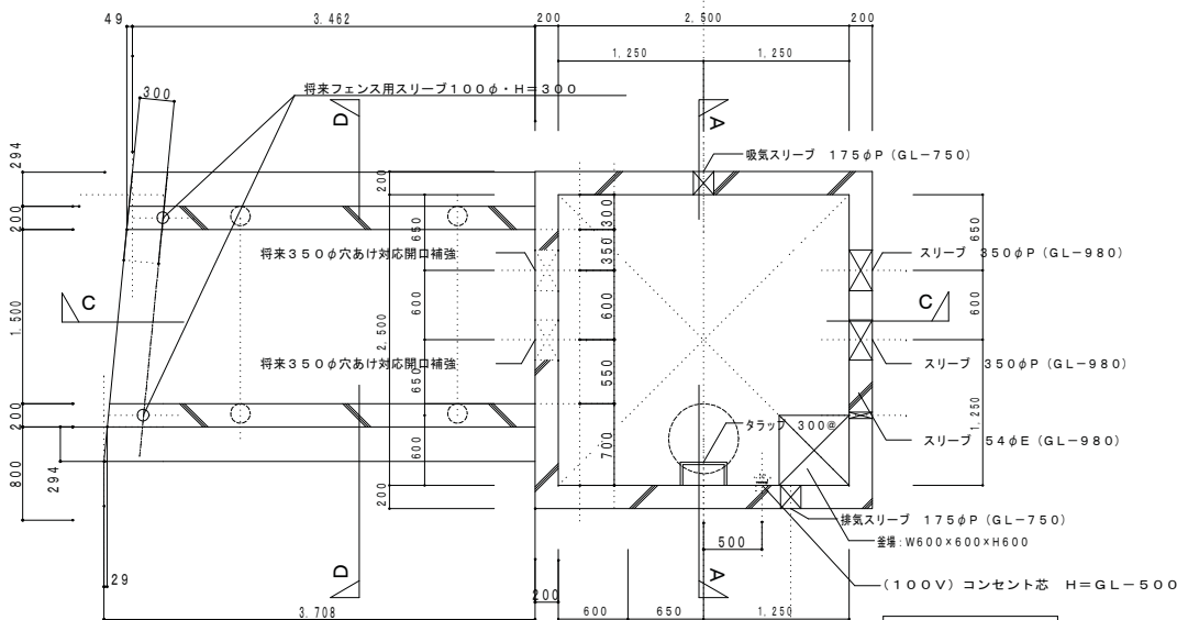
平面図
