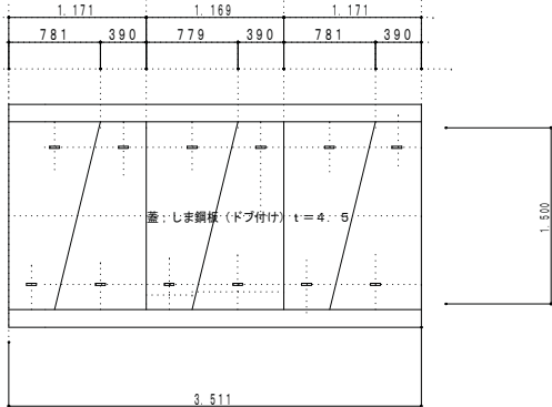
蓋割付図
