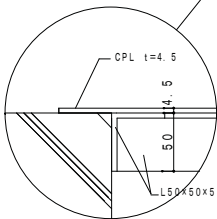
蓋詳細図
