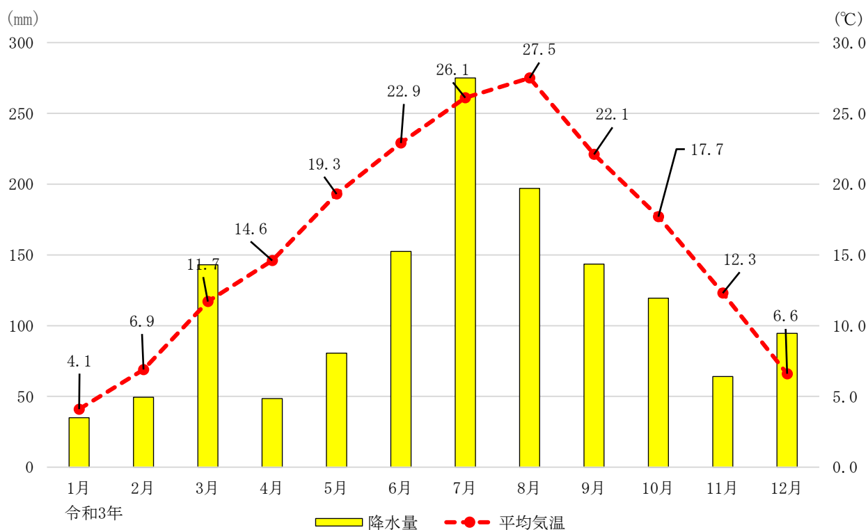
(A-7) 月間降水量と平均気温
