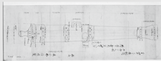
二十四ポンド長銅筒五分一之図(小川家文書)
