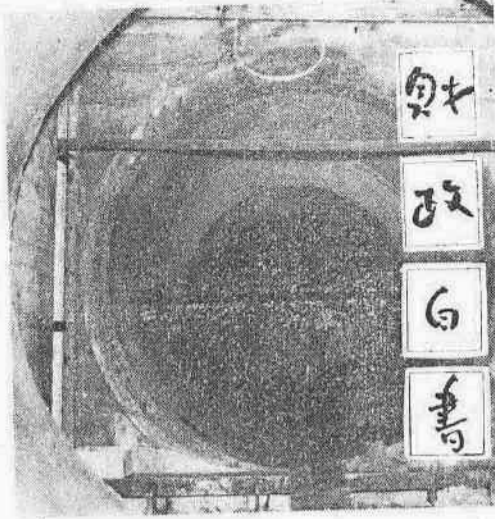
写真は完成した川越・狭山工業団地の下水道内部
